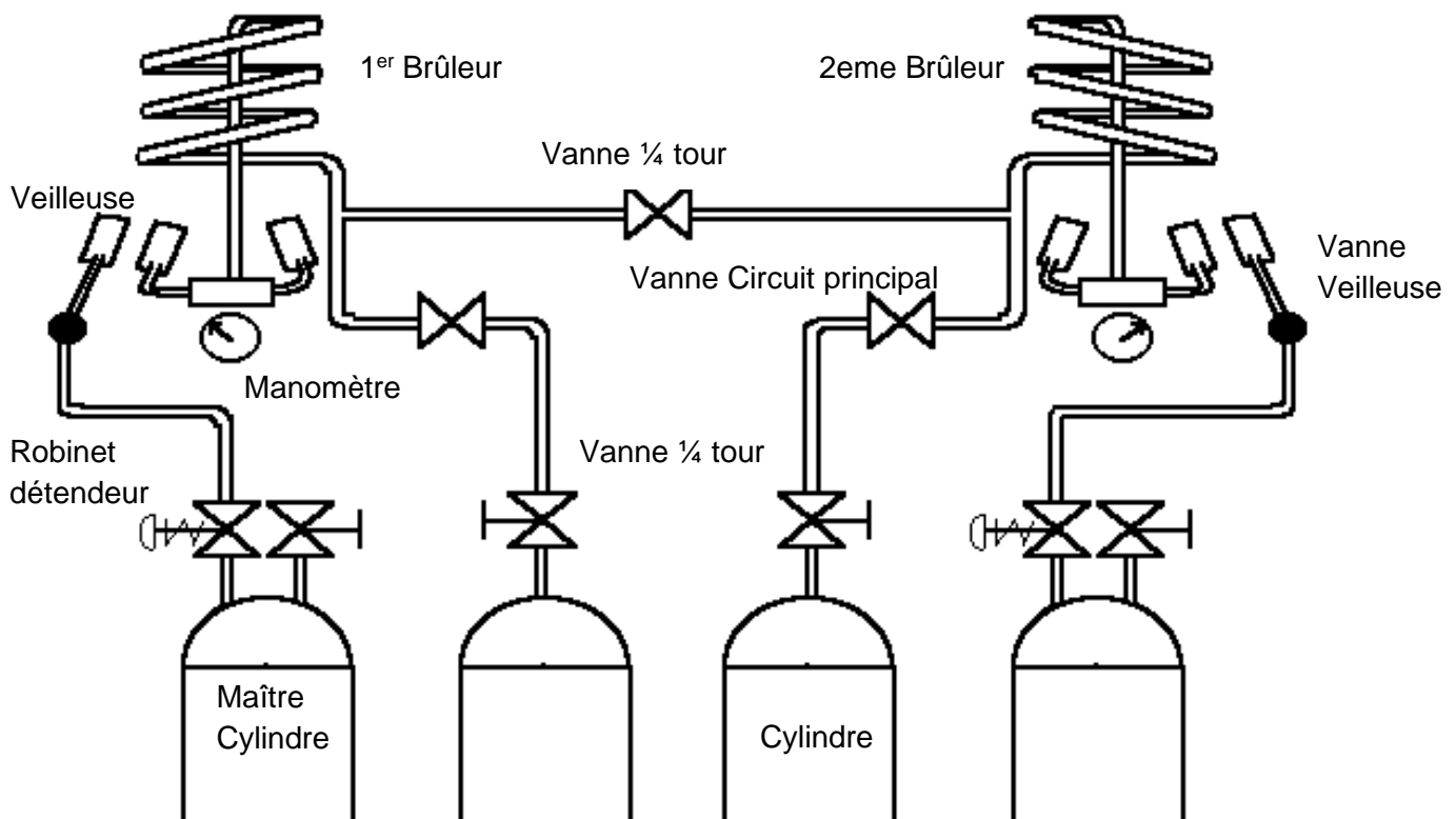
Figure 1 : Montage tous types de brûleur avec veilleuse en phase gazeuse
